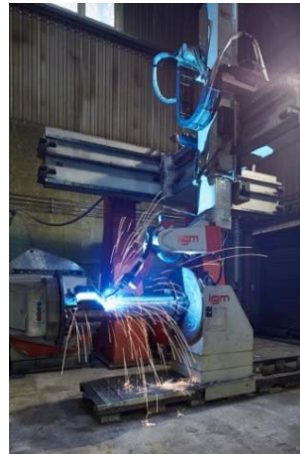
Bild 6: Bei mehrlagigem Schweißen gibt der Einsatz von Schweißrobotern in Korntal-Münchingen und Nördlingen die Gewissheit absolut gleichmäßiger und fehlerfreier Schweißnähte.
